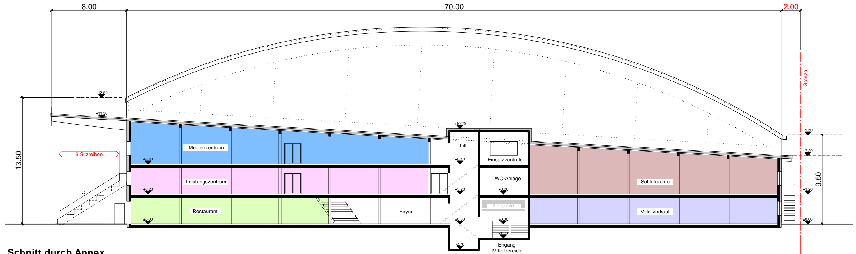
Schnitt durch Annex
